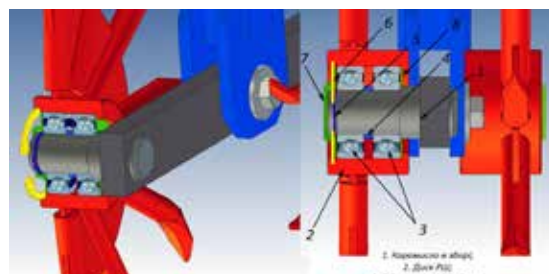
Підшипниковий вузол робочого органу ротаційної борони STEП РШ.
